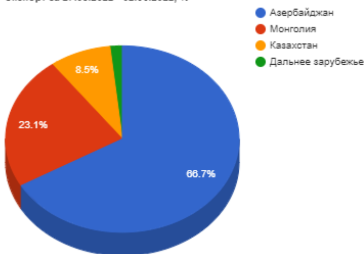
Экспорт за 27.05.2022 - 02.06.2022, %
