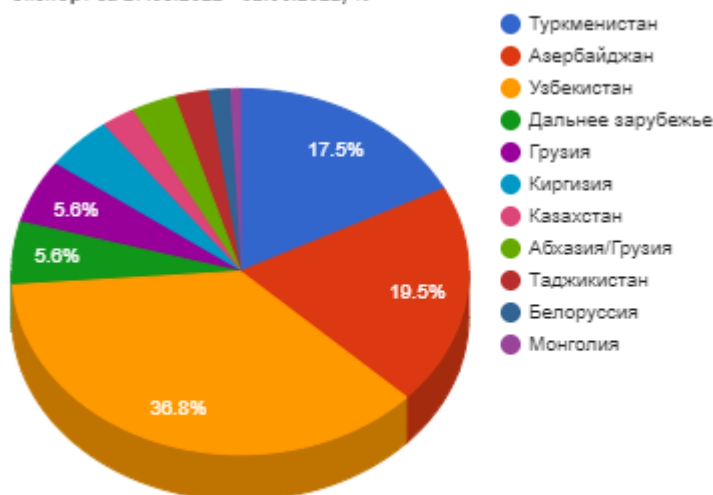
Экспорт за 27.05.2022 - 02.06.2022, %
